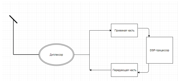
Рис. 1. Блок-схема приемопередатчика СШП
