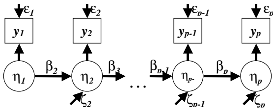
Рис. 3. Однофакторная симплекс-модель
