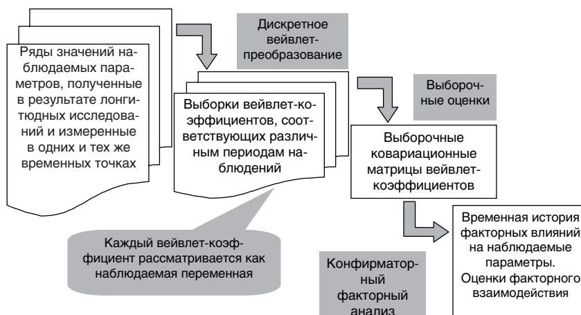
Рис. 1. Основные этапы анализа
