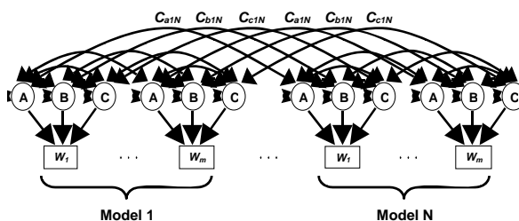
Рис. 7. Изучение факторных влияний в различных условиях: одновременный анализ различных групп моделей. C_{***} – ковариации между факторами
