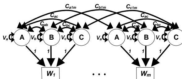
Рис. 6. Модель дисперсионных составляющих, представленная путевой диаграммой
