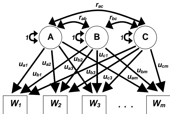
Рис. 5. Модель путей коэффициентов, представленная путевой диаграммой
