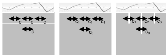
Рис. 9. Примеры различных способов уменьшения числа свободных ковариаций в модели для обеспечения ее переопределенности в случае 8-точечной временной реализации исследуемого параметра
