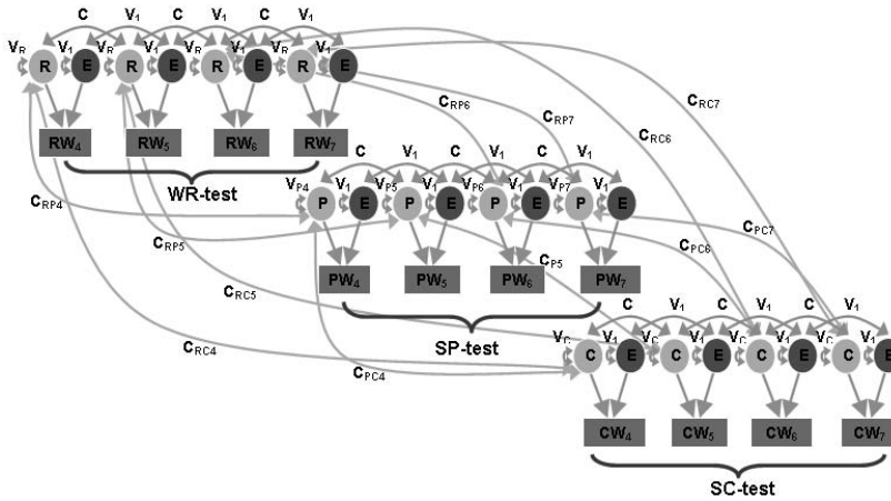
Рис. 11. Модель для исследования двуязычного фонологического восприятия речи у американских школьников: воздействия основных видов фонологического восприятия представлены факторами R, P и C, а связанные с ними искажения, обусловленные несовершенством процедуры исследования – факторами E_R , E_P и E_C . V_* – дисперсии, C_{**} и C_{***} – ковариации между факторами
