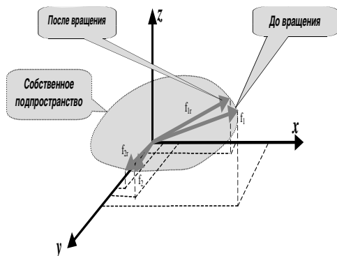
Рис 10. Пример: вращение базиса (f_1, f_2) собственного двухмерного подпространства с целью получения наибольшего соответствия между новыми направлениями координатных осей (f_{1r}, f_{2r}) собственного подпространства и осями исходного трехмерного базиса
