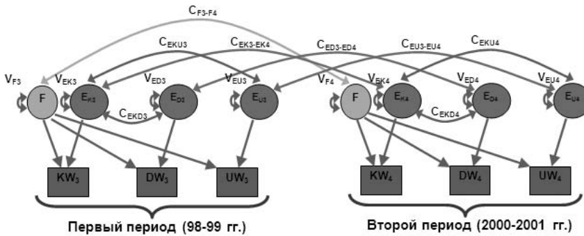
Рис. 12. Модель для выявления общего фактора, влияющего на социально-экономические показатели в различных странах мира: общий фактор обозначен как F, а специфичности переменных K (индекс коррупции), D (индекс Джинни) и U (количество убийств) – как E_K , E_D и E_U . V_F^* – дисперсии общего фактора, V_{E^{**}} – дисперсии факторов ошибок, C_{E^{***}} – ковариации факторов ошибок в одинаковых периодах, C_{E^{**}***} – ковариации факторов ошибок в разных периодах, C_{F_3-F_4} – ковариация фактора F в разных периодах
