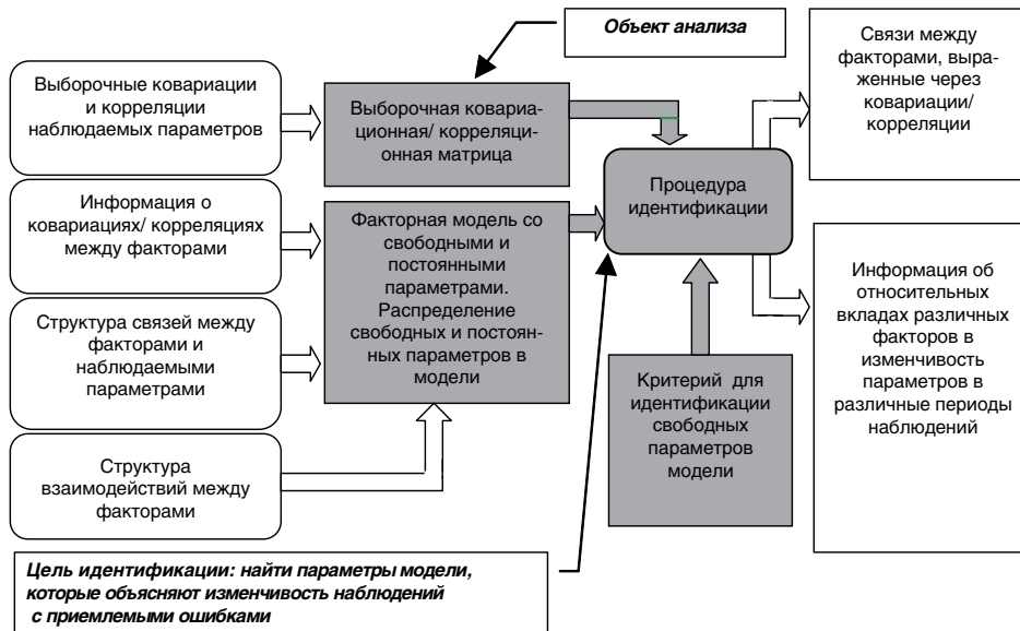
Рис. 2. Основные компоненты конфирматорного факторного анализа. (В случае нескольких типов наблюдаемых случайных процессов для вейвлет-коэффициентов формируется смешанная ковариационная матрица)
