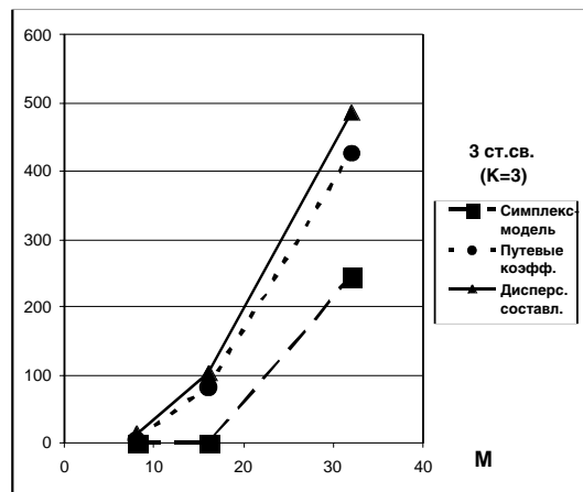
Рис. 8. Степень переопределенности (число степеней свободы) трехфакторной модели ( K=3 ) как функция длин временных реализаций ( M )
